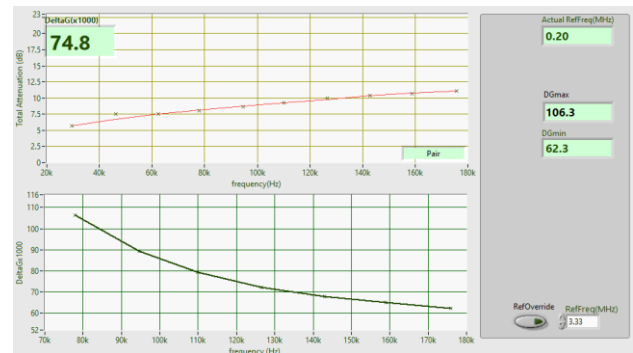
Fig. 5 DeltaG Indicator
